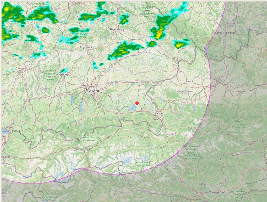
Regenradar · Karte © OpenStreetMap · Radardaten DWD
